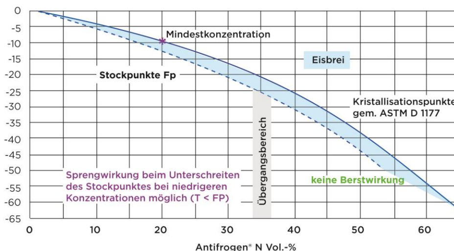
Diagramm 1: Frostsicherheit von Antifrogen® N
