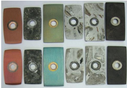
Bild 1: Metallprüfkörper nach ASTM D 1384 (336 h bei 88 °C, 6 l/h Luft) Monoethylenglykol (MEG) ohne Inhibitoren/ ASTM-Wasser (1:2 v/v)
